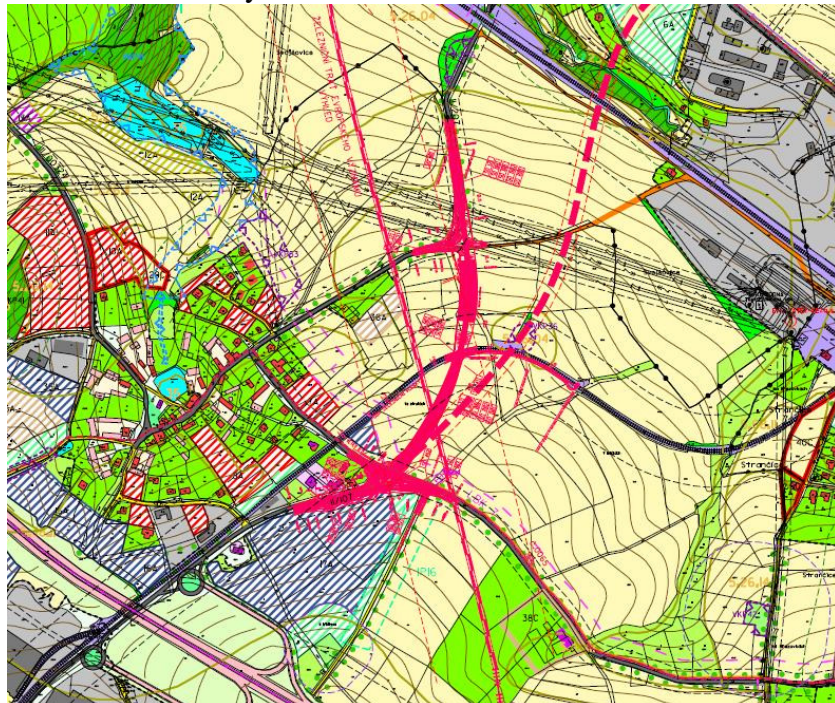
Výřez z dokumentace obchvatu
